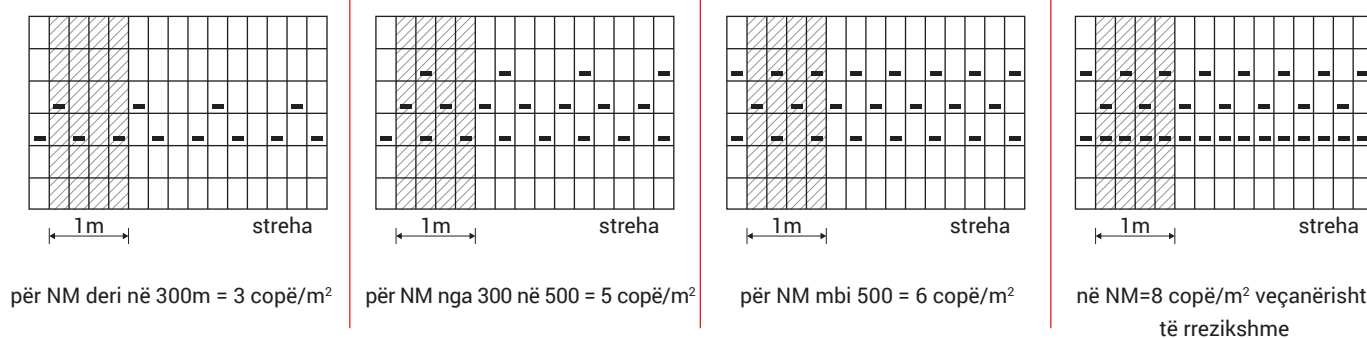
DIAGRAMI I INSTALIMIT TË MBROJTËSES NGA BORA
